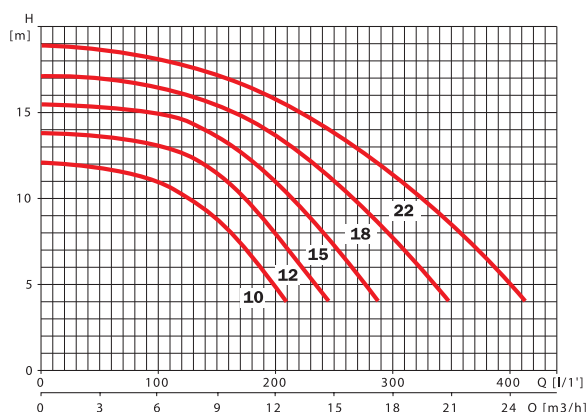
Courbes hydrauliques
