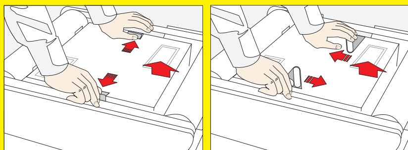
ALETTE DI BLOCCO
