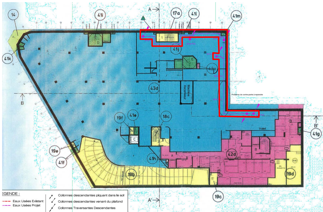
Plan Sous-Sol-1
