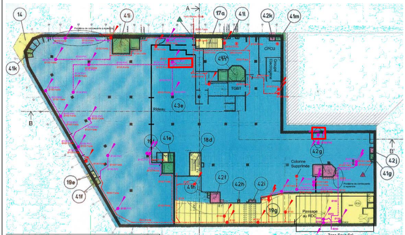
Plan Sous-Sol-1
