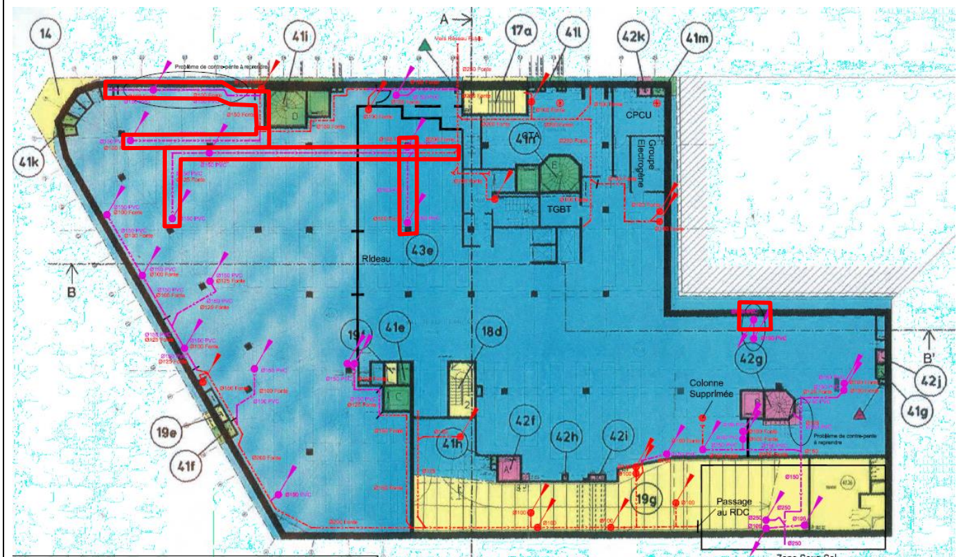
Plan Sous-Sol-1
