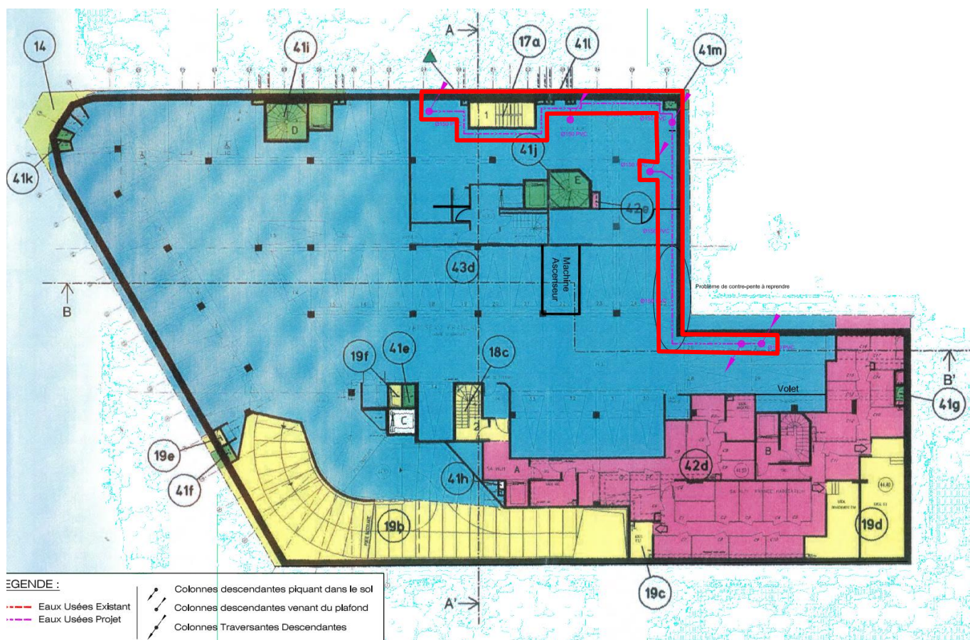
Plan Sous-Sol-1
