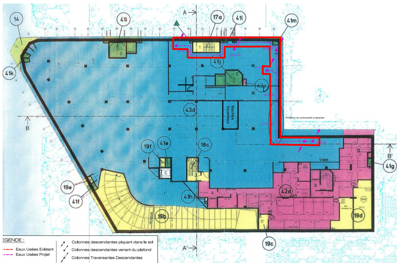
Plan Sous-Sol-1
