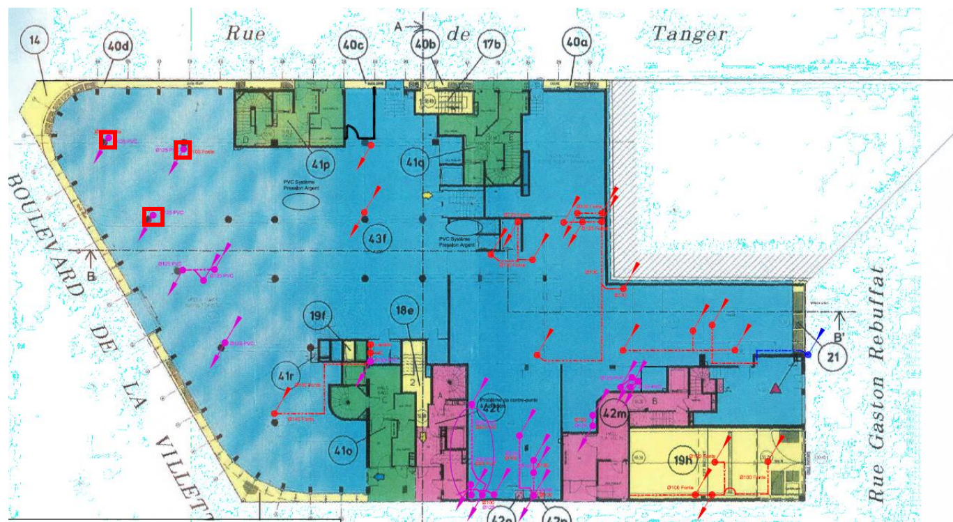
Plan Rez-de-Chaussée
