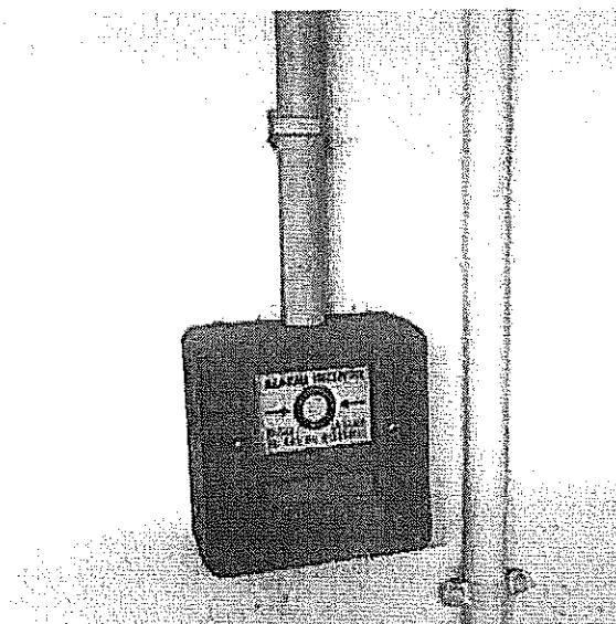
Déclencheur manuel Niveau R-3
